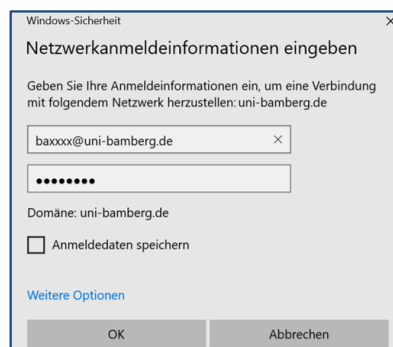
Abbildung 3: Netzwerkanmeldeinformationen eingeben
